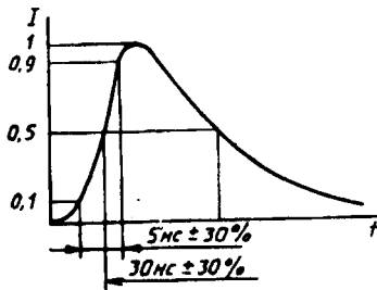
Рисунок Г.2 — Форма волны
